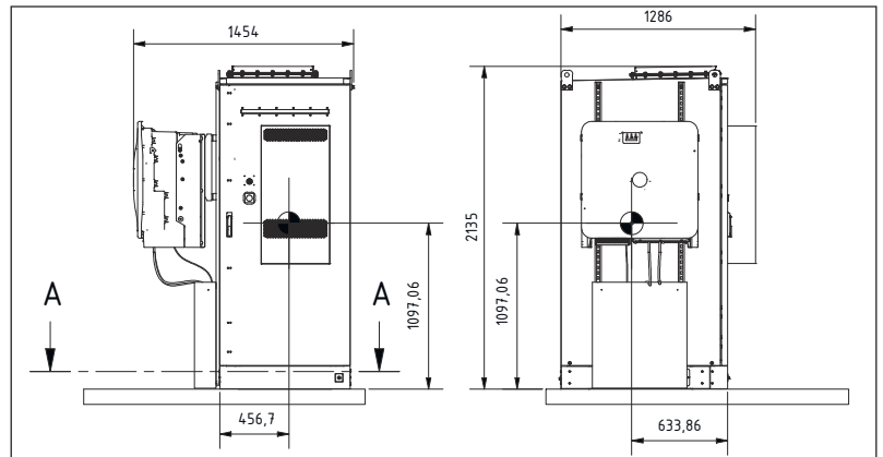
Abb. 15: Empfohlene minimale Fundamentflächen [mm]
