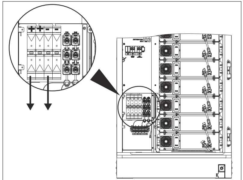
Abb. 23: Übersicht DC-Anschluss Hauptschrank
