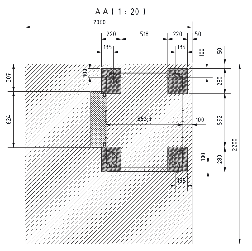
Abb. 16: Flächenansicht [mm]
