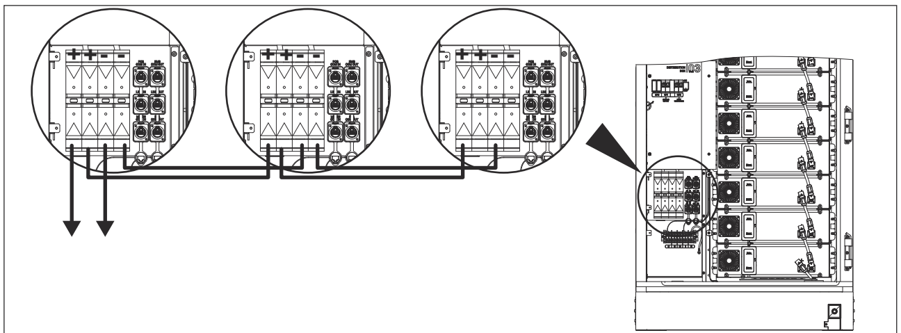
Abb. 24: Übersicht DC-Anschluss mit Erweiterung
