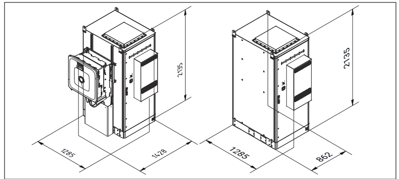
Abb. 9: Maße mit Batteriewechselrichter und Ersatzenergiespeicher [mm]
